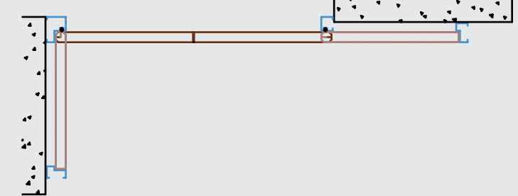
예5) 양개 좌 90°, 우 180° 열리는 문
