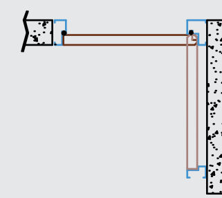
예1) 우힌지 편개 90° 열리는 문
