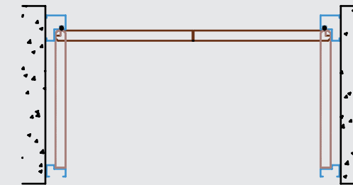
예4) 양개 180° 열리는 문
