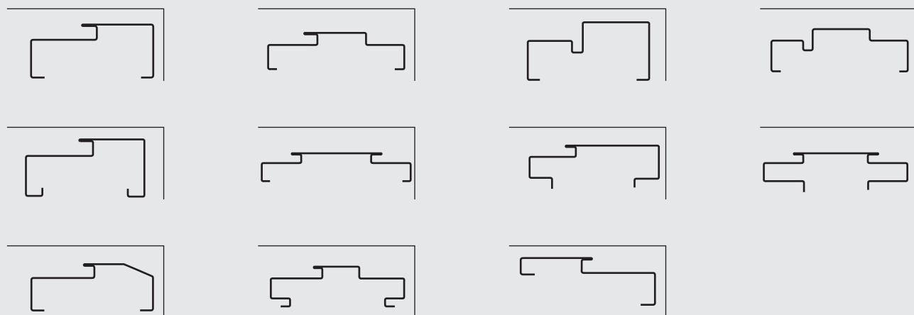
프레임단면도
