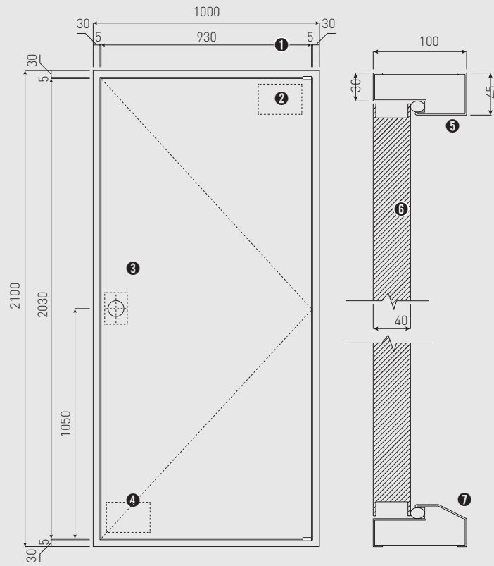
| 입면 상세도 | 수직 단면 상세도
